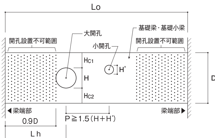
【大開孔位置の規定】
