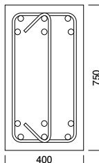
■ 一般部断面
