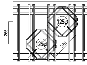
ダイヤレンNS S10×3枚 S筋 (4組3-S13) せん断補強筋 (3-S13 @115)
