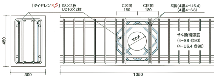
■ 一般部断面
