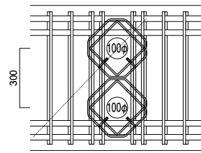
ダイヤレンNS S10×2枚 S筋 (4組3-S13) せん断補強筋 (3-S13 @115)
